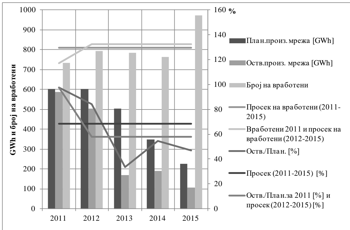
Дијаграм 1 Производство на ЕЕ и вработеност во РЕК Осломеј во периодот 2011-2015 год.
